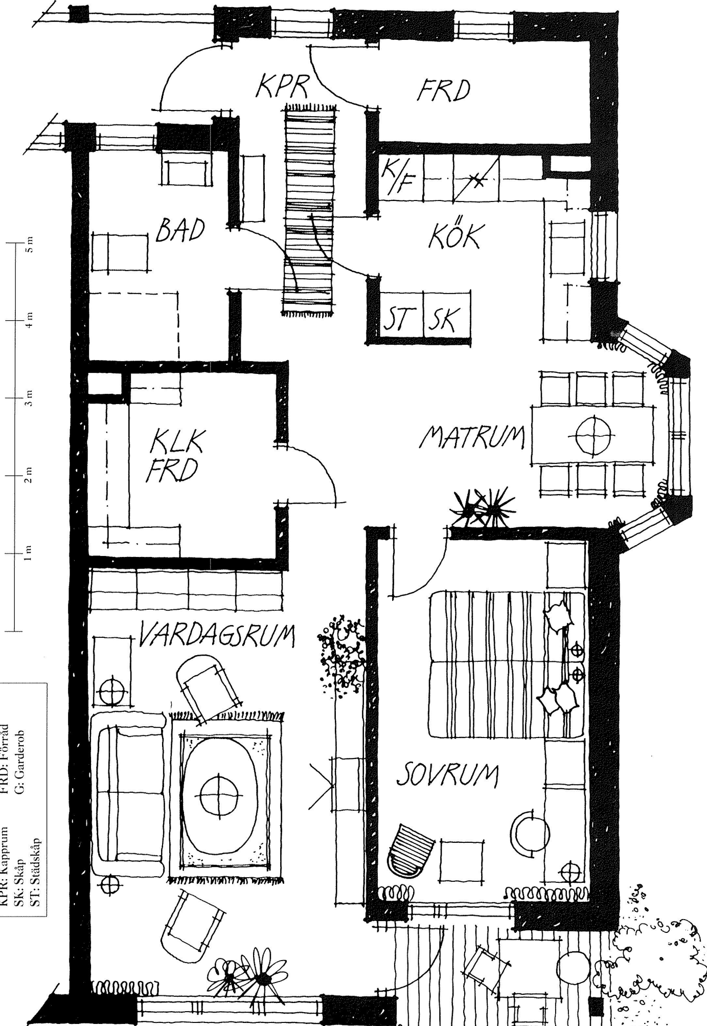
Bottenplan Skala 1:50 UTEPLATS
